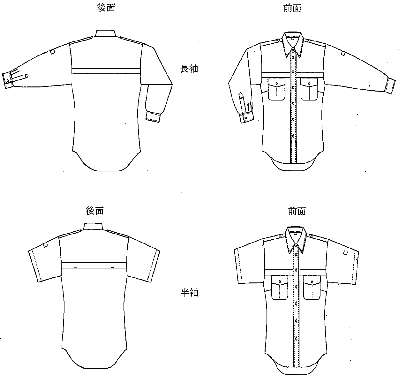
图10 夏服上衣
